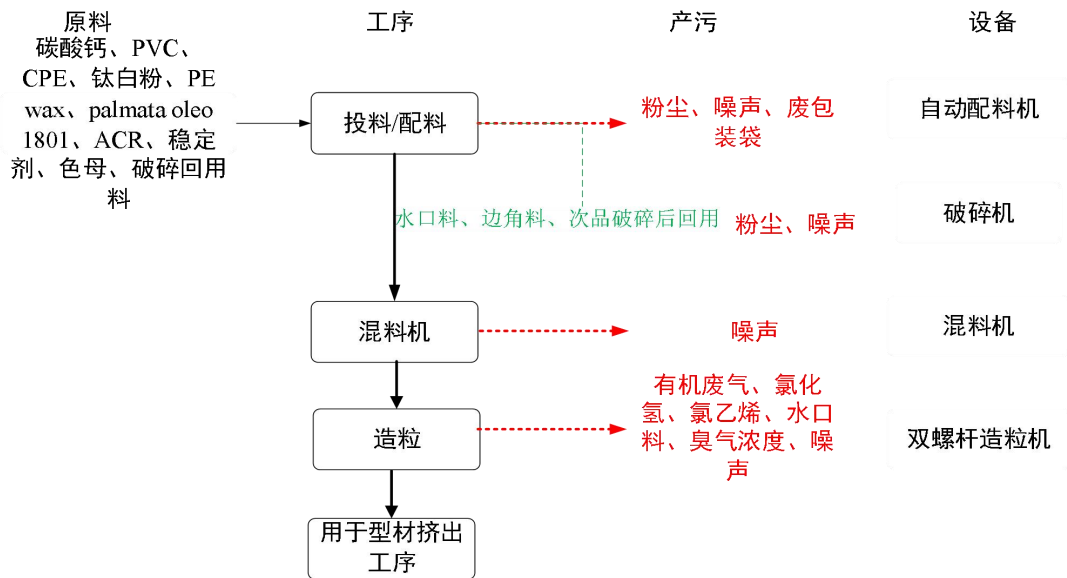
图 2-5 造粒生产工艺流程图
