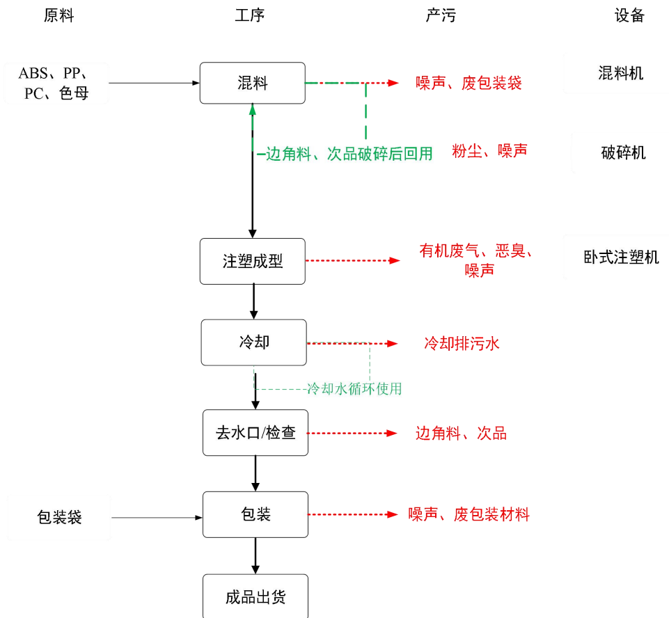
图 2-4 塑胶制品生产工艺流程图
