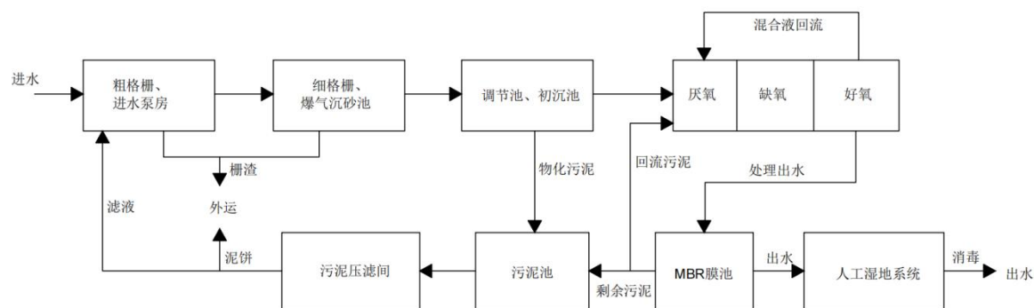
图 4-2 鹤山工业城鹤城共和片区污水处理厂污水处理工艺流程图
