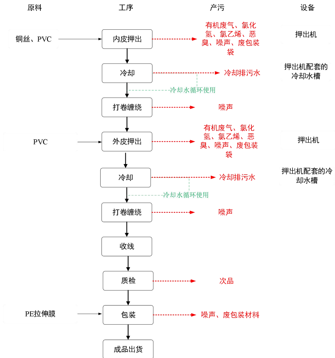
图 2-2 电线生产工艺流程图
