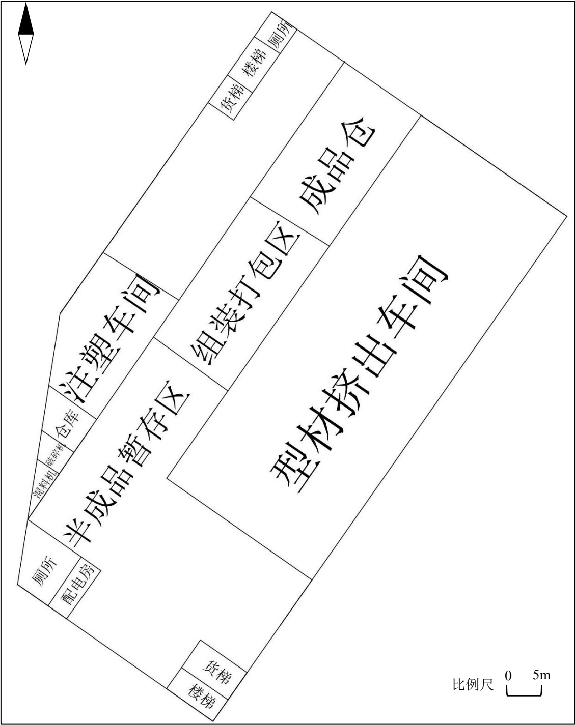
附图 4c 项目 1#厂房一层平面布置图
