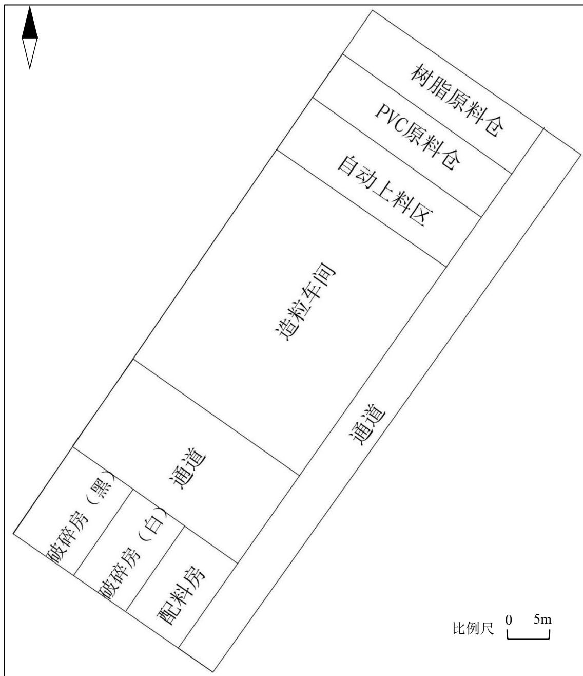
附图 4f 项目 2#厂房平面布置图
