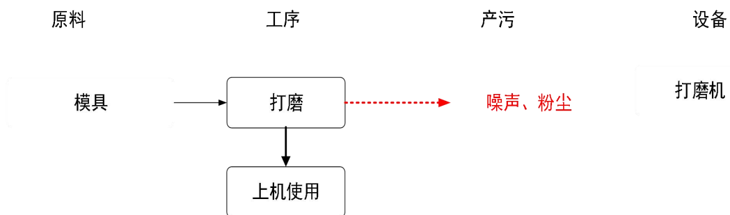
图 2-8 模具打磨工艺流程图
