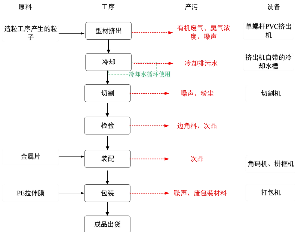
图 2-6 塑料型材生产工艺流程图
