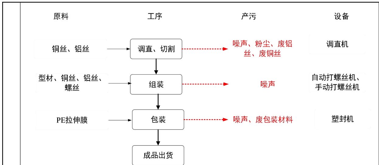
图 2-7 轨道条生产工艺流程图
